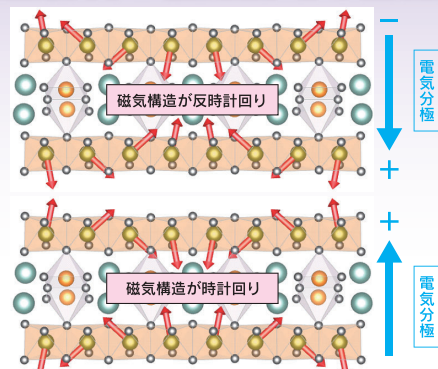
マルチフェロイック磁性材料の結晶・磁気構造と分極の関係の解明
